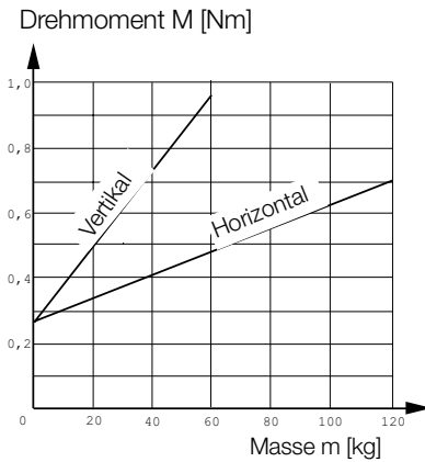
Baugröße OSP-E32SB, Steigung 5 mm Beschleunigung 2 m/s 2
